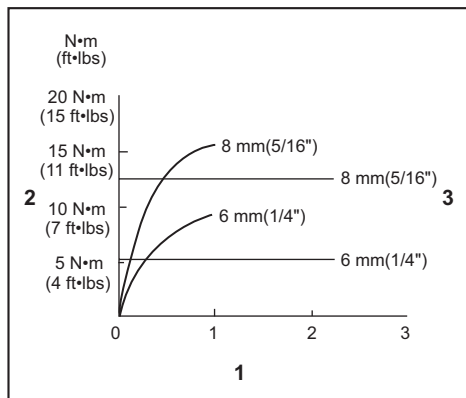
1. Tiempo de apriete (segundos) 2. Torsión de apriete 3. Torsión de apriete apropiada correspondiente al diámetro de cada perno
